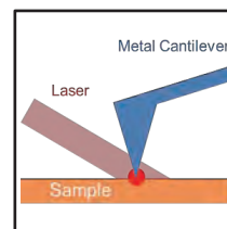
TERSの模式図
