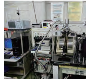
広帯域磁気光学効果エネルギー依存性評価機
