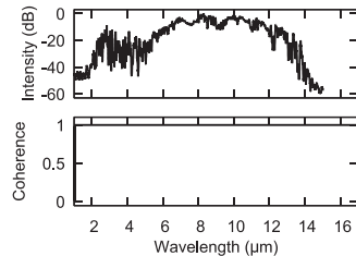
高コヒーレント中赤外スーパーコンティニューム光の特性
