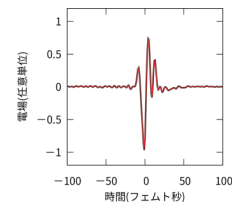
開発された計測技術によって測定された超短光パルスの電場波形
