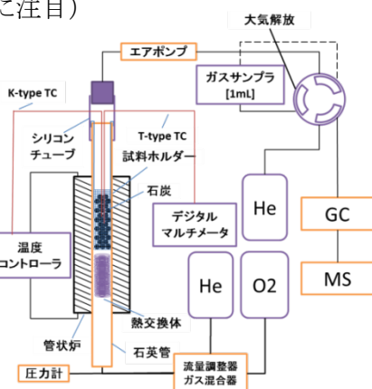
バイオマスのガス化実験 (GC-MS等による生成物分析、低温での反応機構)
