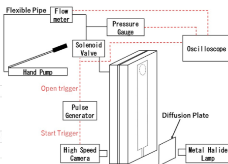
高粘度液体の噴霧実験 (キャビテーション発生条件等)
